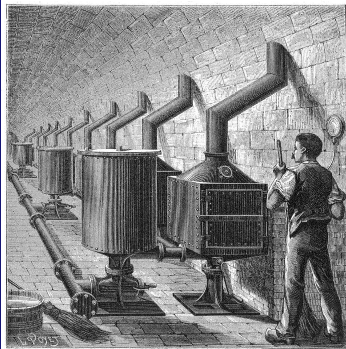
Fig. 1. — Vidange pneumatique. — Vue d'ensemble des appareils récepteurs de la caserne de la Pépinière, à Paris.
